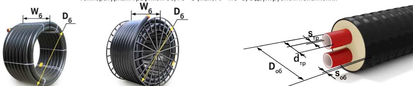
ТВЭЛ-ПЭКС-2-К. Номенклатура, размеры для транспортировки и монтажа
