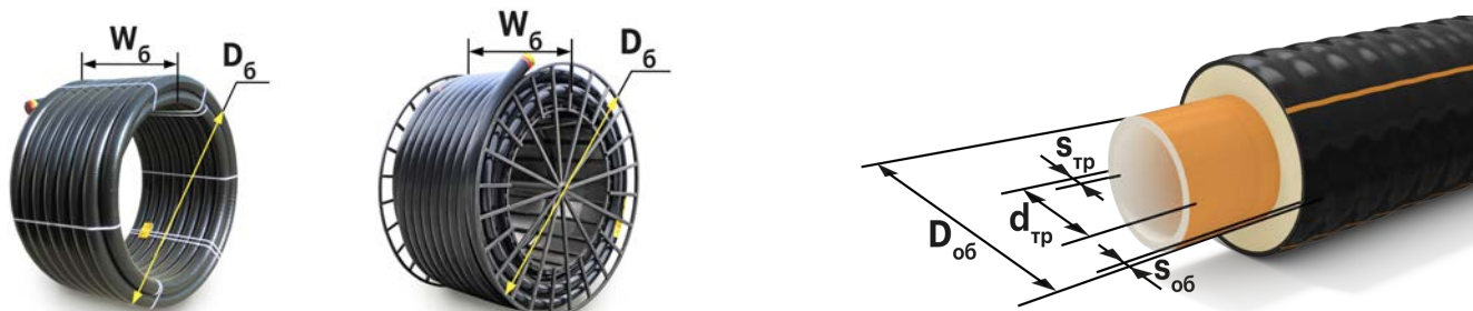
ТВЭЛ-ПЭК-115-К. Номенклатура, размеры для транспортировки и монтажа
