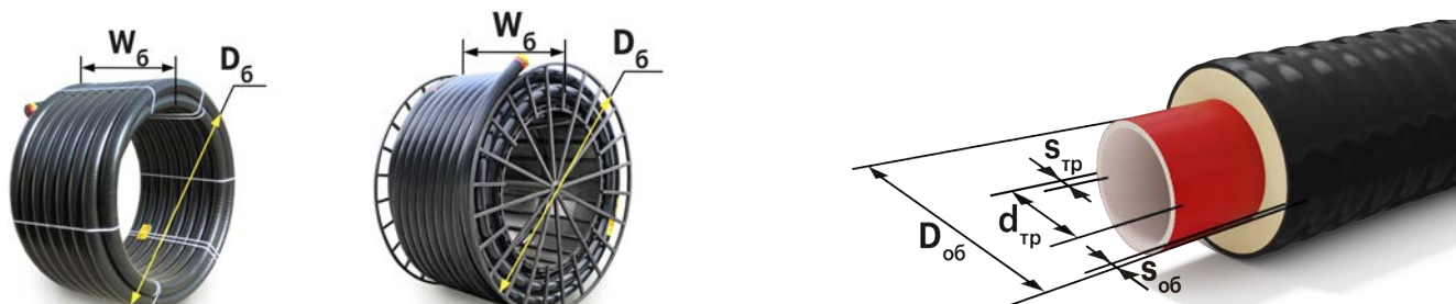
ТВЭЛ-ПЭКС-К. Номенклатура, размеры для транспортировки и монтажа
