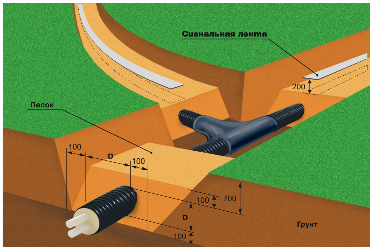
Профиль траншеи для трубопроводов ТВЭЛ-ПЭКС, размеры в мм
