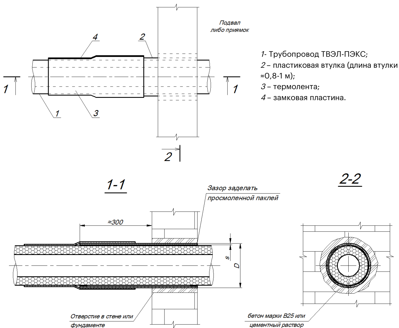
Рис. 22. Узел прохода через стену
