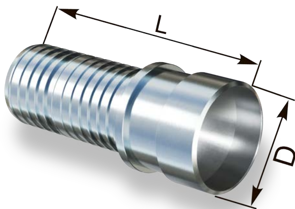
Рис.13. Фитинг компрессионный под сварку
