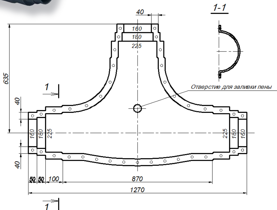
Рис. 15. Кожух для изоляции тройника (для диаметров оболочек 160-225)
