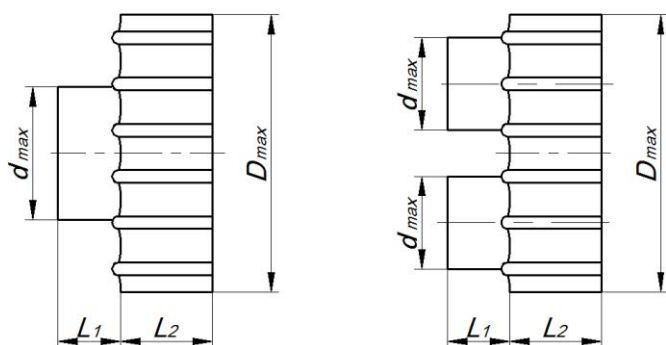
Рис. 21. Термоусаживающаяся заглушка
