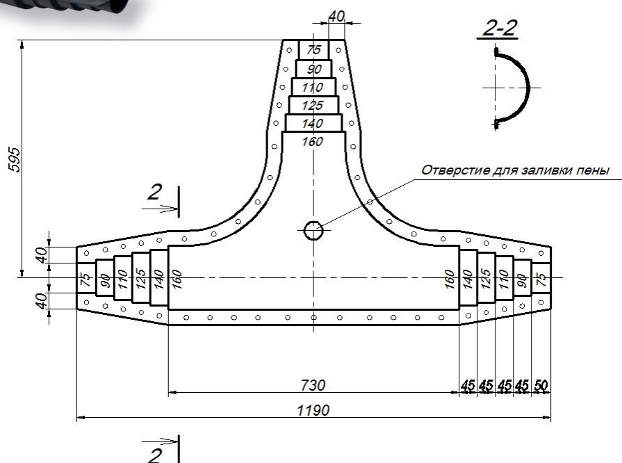
Рис. 16. Кожух для изоляции тройника, универсальный (для диаметров оболочек 90-160 мм)
