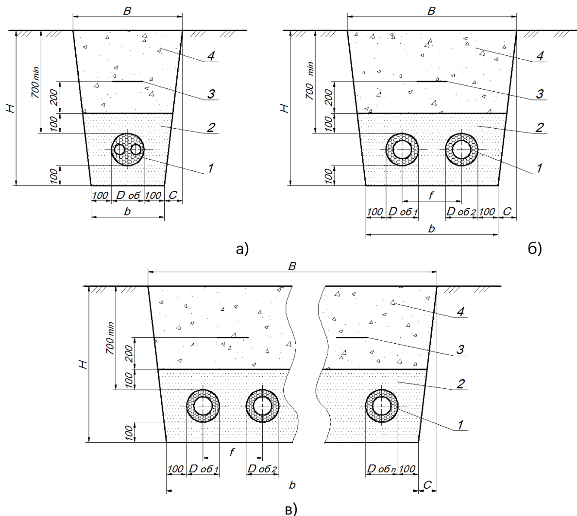
Рис. 23. Размеры траншеи (а - однотрубная прокладка, б - двухтрубная прокладка, в - многотрубная прокладка)
